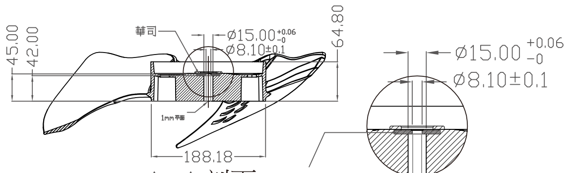
A-A 剖面 華司 \varnothing 8 \times \varnothing 38
